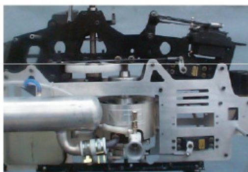
NR-12Hヘリ搭載
