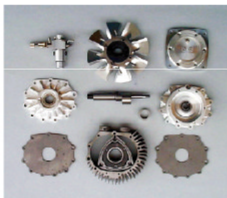
NR-12H構成部品
